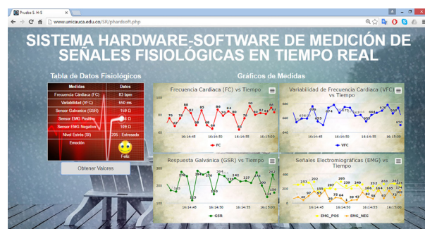
Figure 11. Web interface for monitoring physiological variables and user emotion / Interfaz web para monitoreo de variables fisiológicas y emoción de usuario
