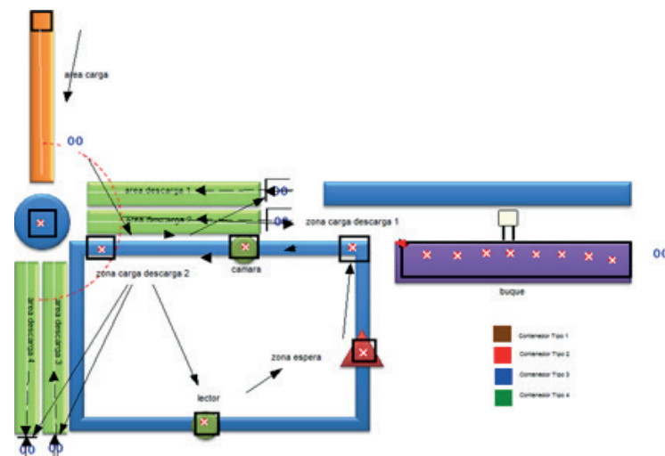
Figura 3. Simulación en ProModel de la práctica 2, asociada a una operación portuaria / Simulation in ProModel® of practice 2, associated with port operations
