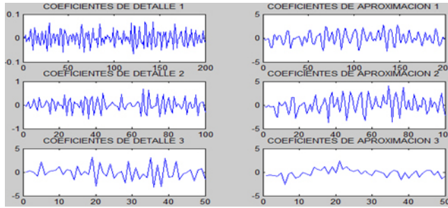
Figura 2. Descomposición Wavelet de tres niveles de una señal de audio
