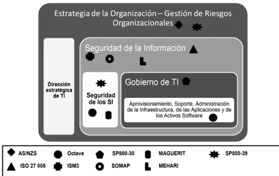
Gráfico 3. Alineamiento de los estándares sobre GRCSI con las actividades del negocio
